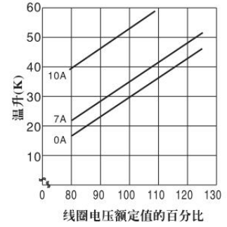
线圈温升
